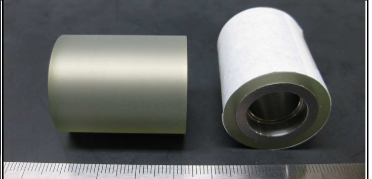
製品番号: SS12U40298ENS 使用用途: Rローラ ローラー寸法 長:35 径:φ28 硬度: 90エステル シャフト寸法 長:35 径:φ①22 ②16 ③14
