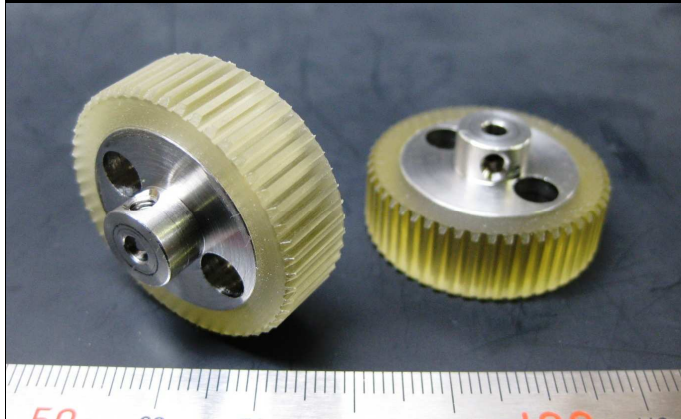
製品番号: SS12U37319ENS 使用用途: Pローラ ローラー寸法 長:10 径:φ30 硬度: 28エステル シャフト寸法 長:10 径:φ① 22 ②9 ③3
