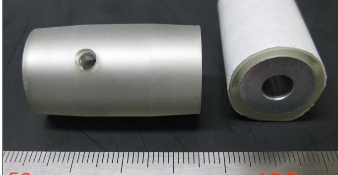
製品番号: SS12U42301ENS 使用用途: Dプーリ ローラー寸法 長:35 径:φ20 硬度: 60エステル シャフト寸法 長:35 径:φ①16 ②6.4
