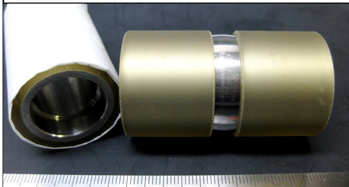
製品番号: SS12U80441LNS 使用用途: HPローラ ローラー寸法 長:55.9 径:φ32 硬度: 35エステル シャフト寸法 長:55.9 径:φ①30 ②26 ③19
