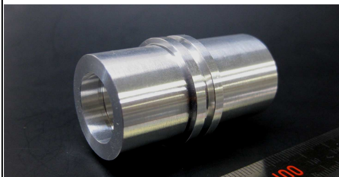
製品番号: SS12M90302ENS S9 寸法: 全長: 46.5 径: \phi ①24 ②22 ③16
