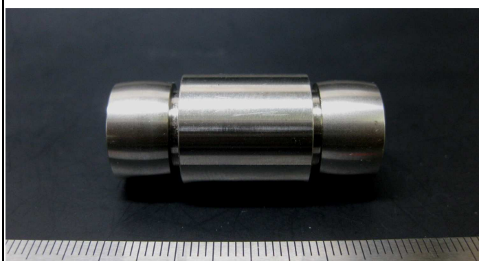
製品番号: SS12M40311LNS SUS303 寸法: 全長: 40 径: \phi ①18 ②16
