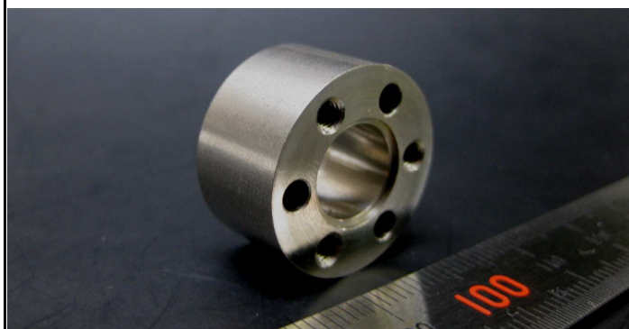
製品番号: SS12M69541ENS SUS303 寸法: 全長: 12 径: \phi ①22 ②11.4 ③10
